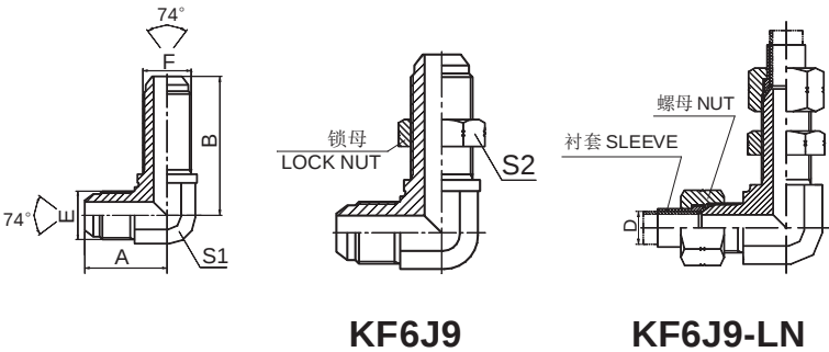
90° JIC MALE 74° CONE BULKHEAD 90° JIC 外螺纹 74° 外锥过板接头
