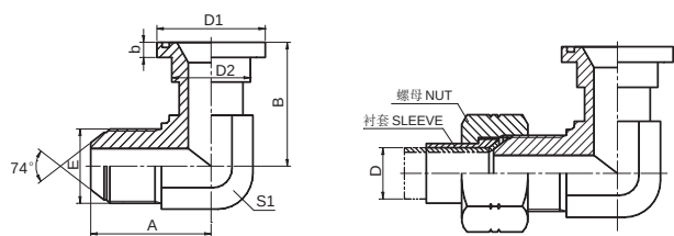
90° 弯美制 JIC 外螺纹 74° 外锥 / 重系列法兰 ISO 6162-2 KF1JFS9 90° ELBOW JIC MALE 74° CONE / S-SERIES FLANGE ISO 6162-2
